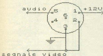
fig. 3: presa standard VCR e monitor (PAL—CCIR)
